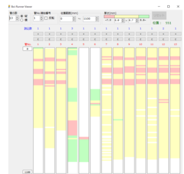
複数の管の厚さを3段階カラー表示 任意の閾値を定めてパネル全体の肉厚を色で表示します。もちろん管1本1本の厚さをグラフ化することも可能です。
