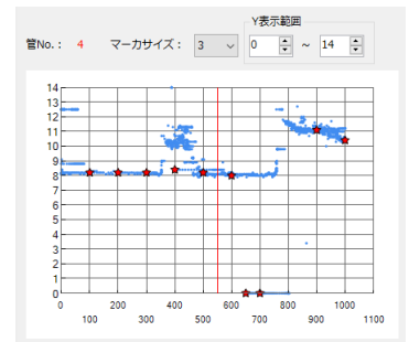
計測結果をその場でグラフ化 計測結果の点群と任意の代表点の厚さを表示します。
