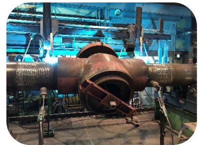
偏心軸の自動肉盛溶接
