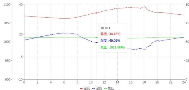
工場の温度・湿度・気圧記録
